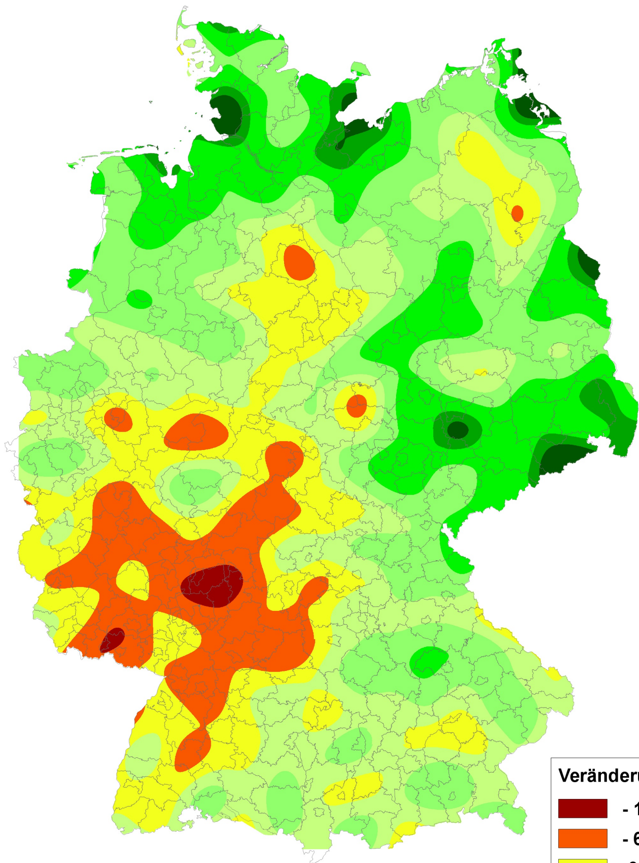
Veränderung des Sommerniederschlag in Deutschland Im Referenzzeitraum 1980 - 2010 gegenüber 1960 - 1990
